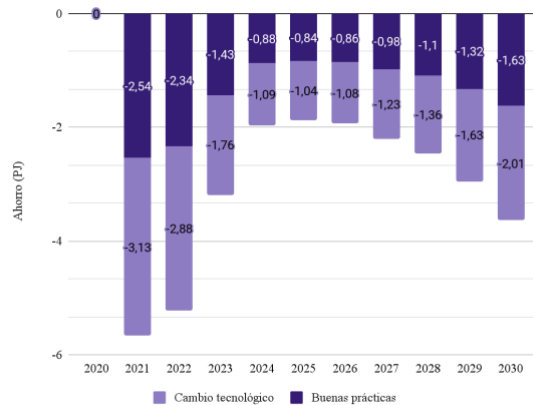
Gráfica 27. Simulación de los ahorros energéticos en el parque termoeléctrico por la adopción de medidas analizadas.
