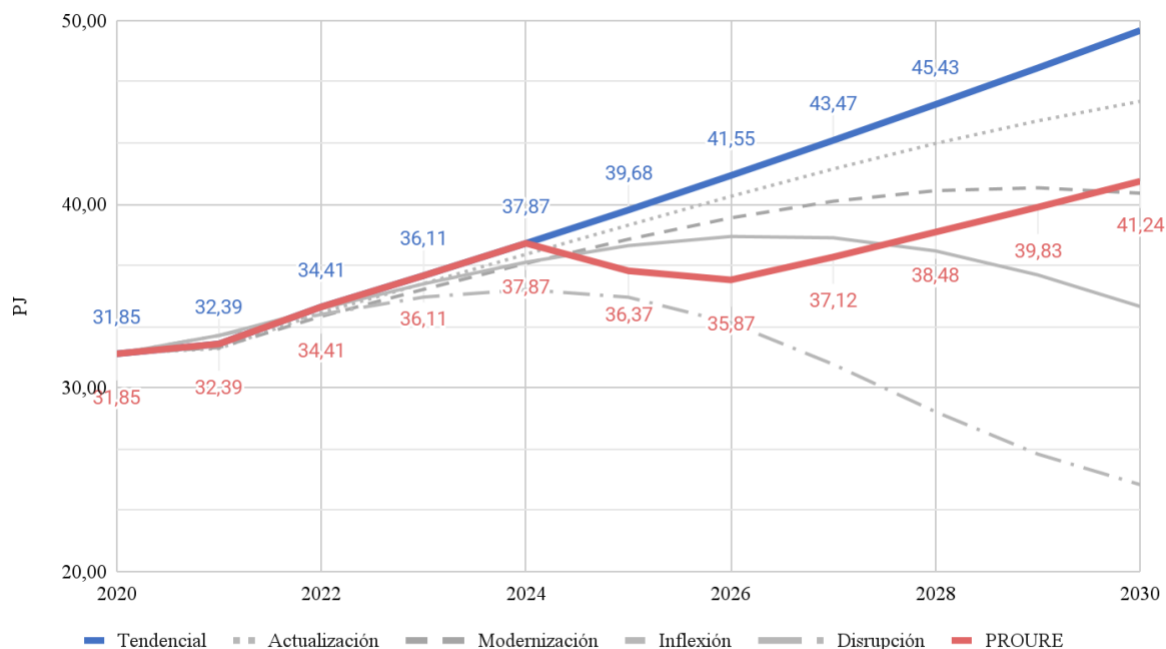
Gráfica 37. Comparación de escenarios de consumo energético para el consumo de aire acondicionado y ventilación en el sector residencial y comercial.
