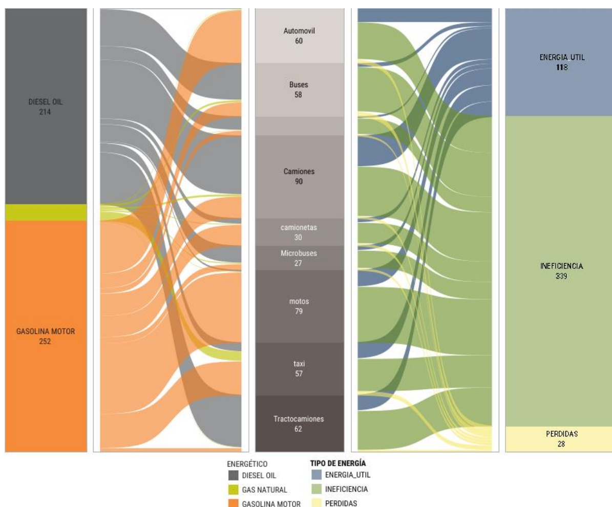
Gráfico 12. Energéticos y usos del sector transporte carretero (energía en PJ)
