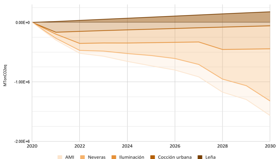
Gráfica 11. Reducción estimada de emisiones de las medidas de eficiencia energética en el sector residencial en el PAI-PROURE
