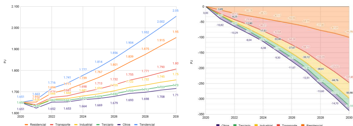
Gráfica 5. Ahorros potenciales en el consumo de energía de las medidas analizadas en el PAI-PROURE 2021-2030 por sector
