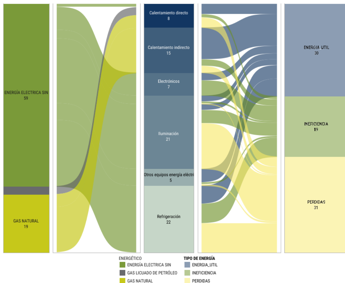
Gráfica 21. Energéticos y usos del sector terciario (energía en PJ)
