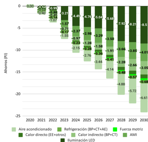
Gráfica 23. Reducción de demanda esperada de las medidas de eficiencia energética en el sector terciario en el PAI-PROURE
