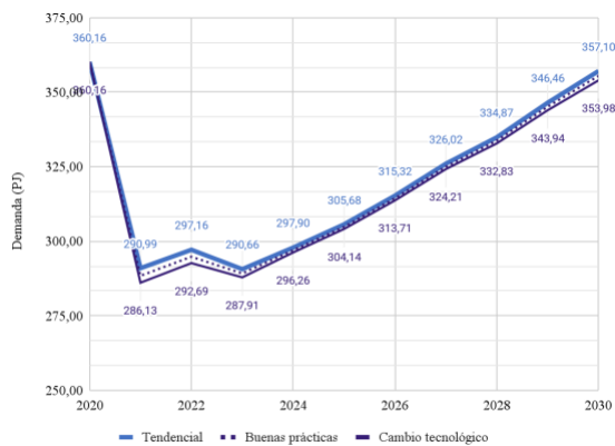
Gráfica 27. Simulación de los ahorros energéticos en el parque termoeléctrico por la adopción de medidas analizadas.
