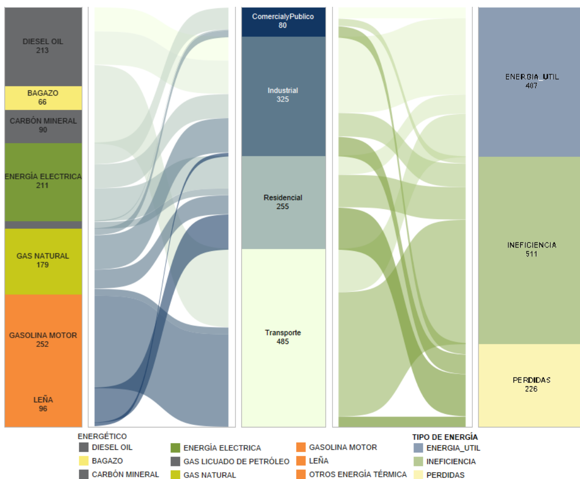
Gráfica 1. Balance de energía útil 2019
