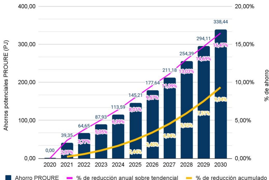
Gráfica 2. Potenciales de eficiencia energética por año PAI-PROURE 2021-2030
