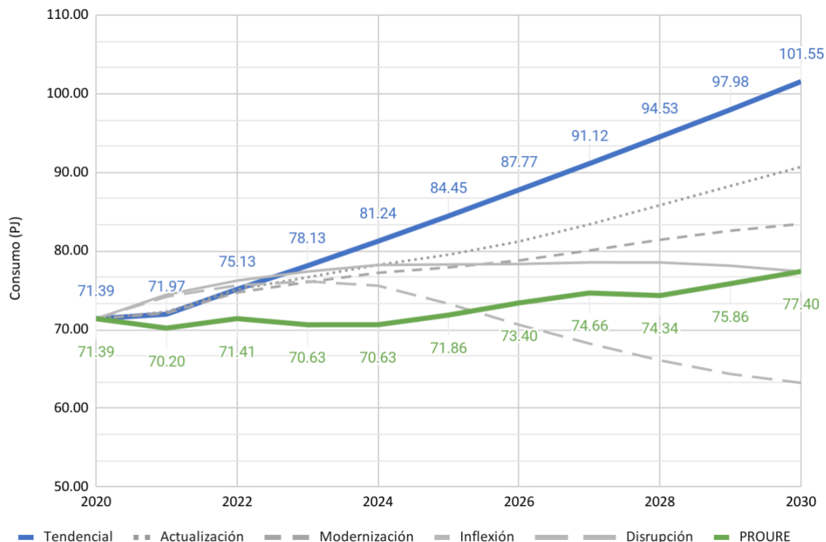
Gráfica 22. Comparación de escenarios de consumo energético para el sector terciario.
