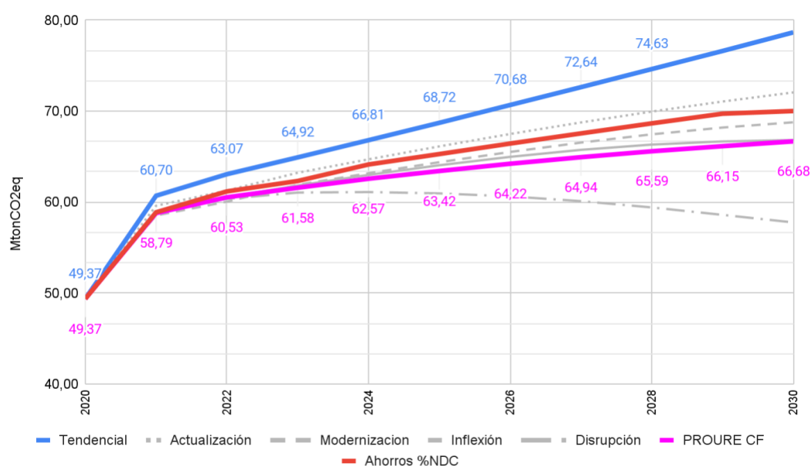
Gráfica 6. Comparación de las emisiones estimadas para el escenario PAI-PROURE 2021-2030 frente al escenario tendencial y los del PEN 2020-2050
