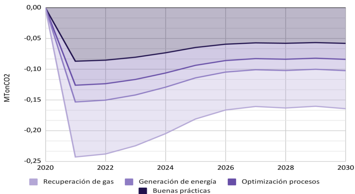
Gráfica 32. Reducción estimada de emisiones de las medidas de eficiencia energética en el sector hidrocarburos en el PAI-PROURE
