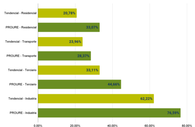
Gráfica 41. Porcentaje de energía útil sobre energía final
