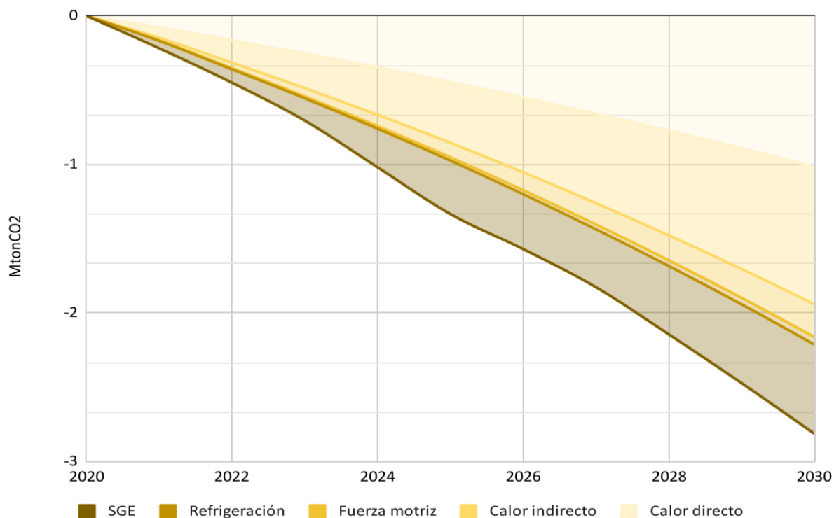
Gráfica 20. Reducción estimada de emisiones de las medidas de eficiencia energética en el sector industrial en el PAI-PROURE
