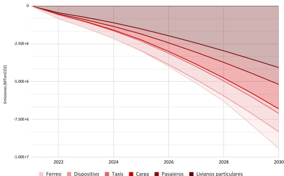
Gráfica 16. Reducción estimada de emisiones de las medidas de eficiencia energética en el sector transporte en el PAI-PROURE
