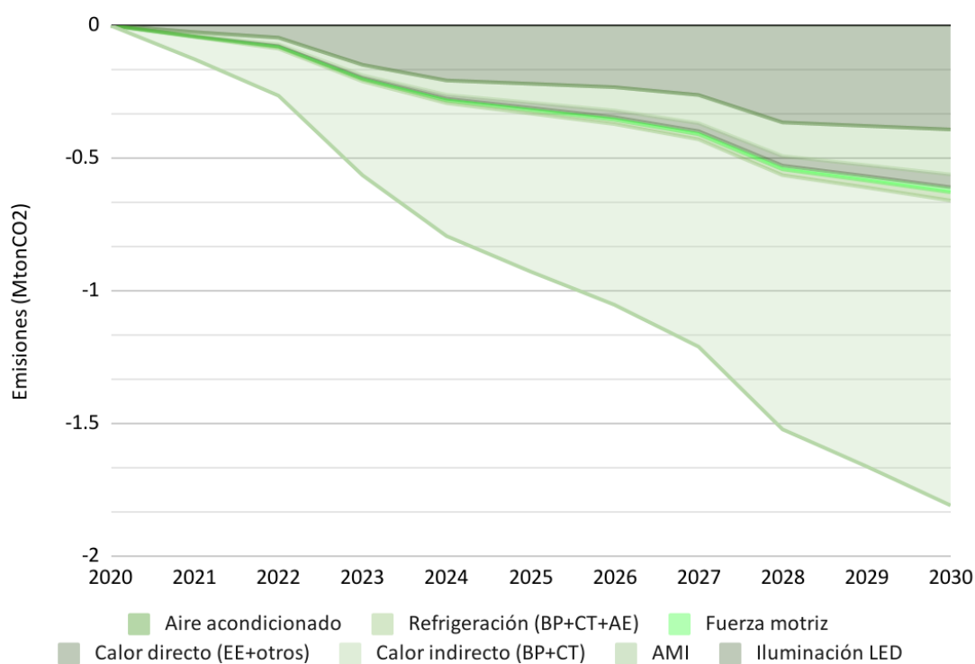
Gráfica 24. Reducción estimada de emisiones esperada de las medidas de eficiencia energética en el sector terciario en el PAI-PROURE
