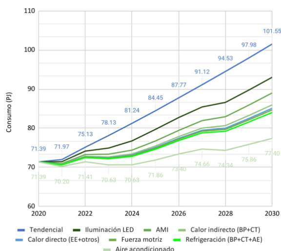
Gráfica 23. Reducción de demanda esperada de las medidas de eficiencia energética en el sector terciario en el PAI-PROURE
