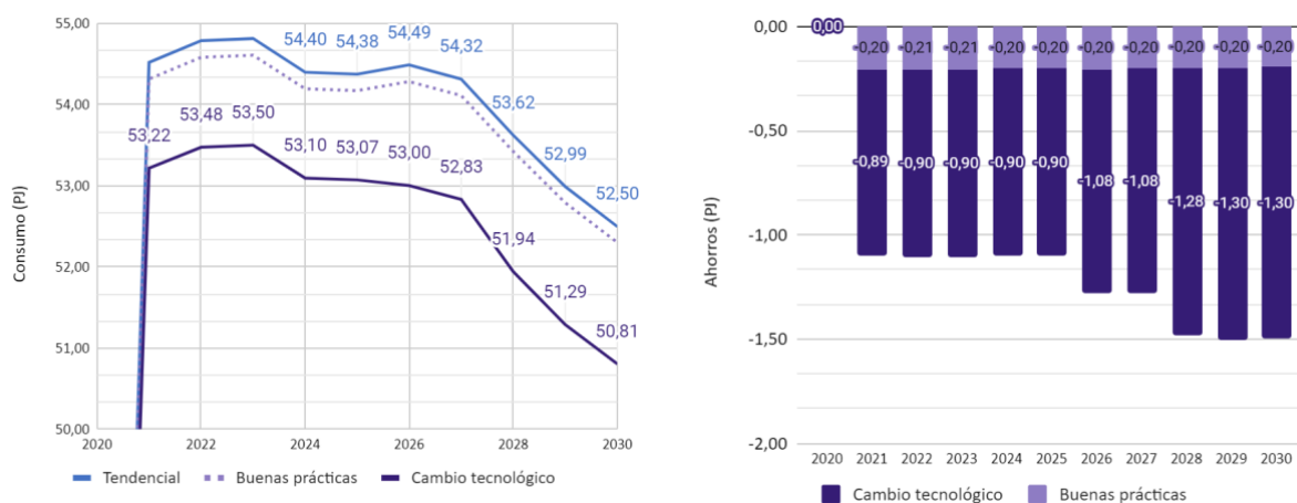
Gráfica 35. Simulación de los ahorros energéticos en el sector minero por la adopción de las medidas analizadas.
