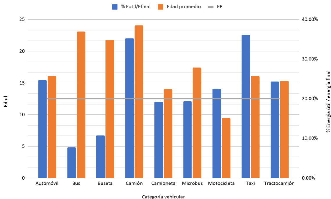
Gráfica 13. Energía útil y edades promedio por categoría vehicular
