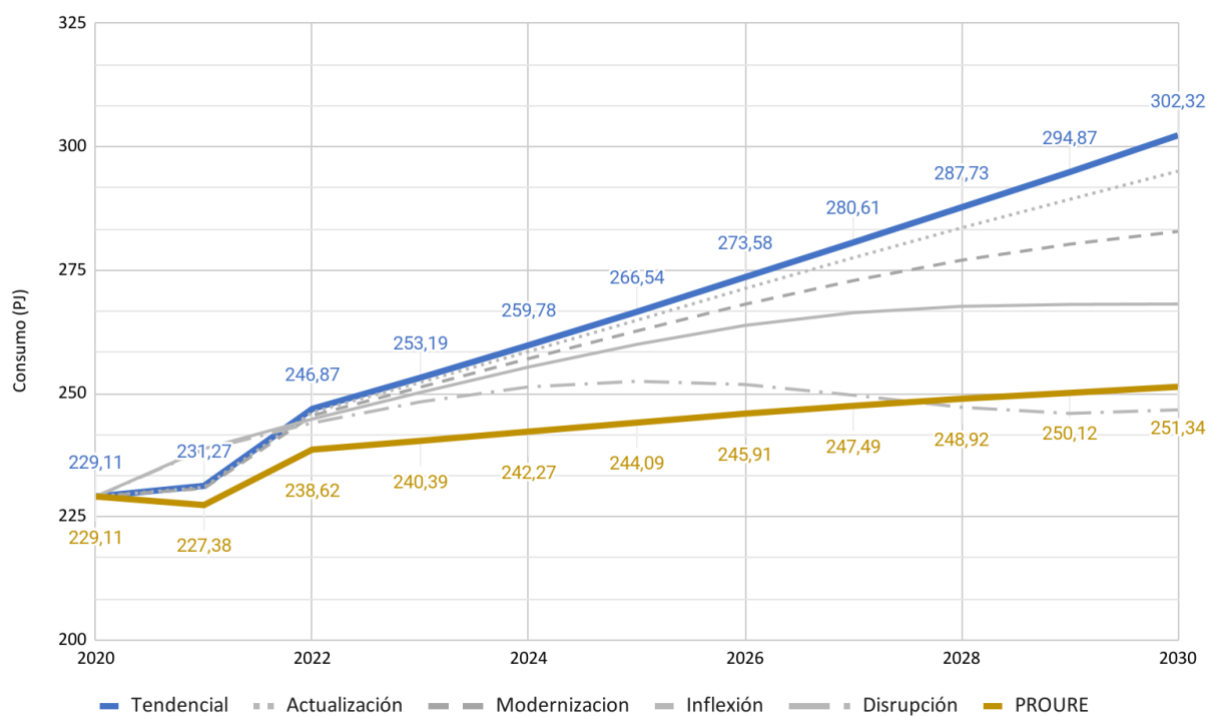
Gráfica 18. Comparación de escenarios de consumo energético para el sector industrial.
