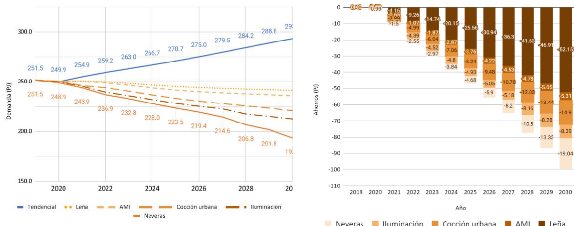
Gráfica 10: Reducción de demanda esperada de las medidas de eficiencia energética en el sector residencial en el PAI-PROURE
