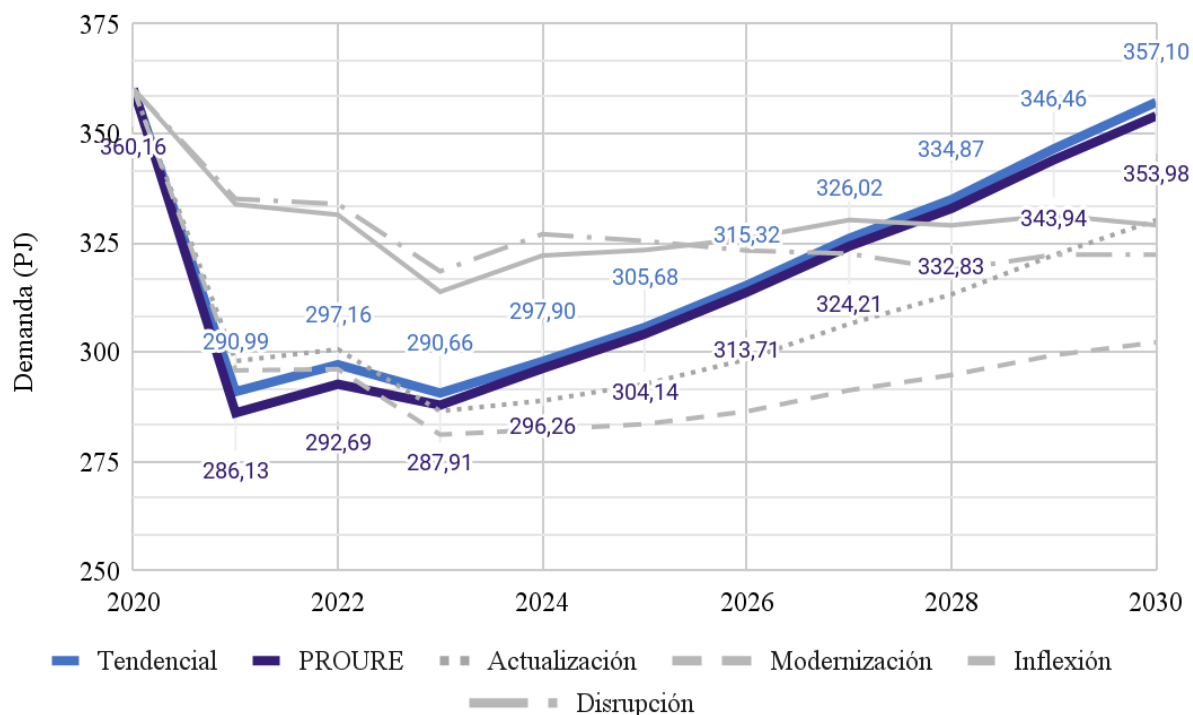
Gráfica 26. Comparación de escenarios de consumo energético para el sector termoeléctrico.
