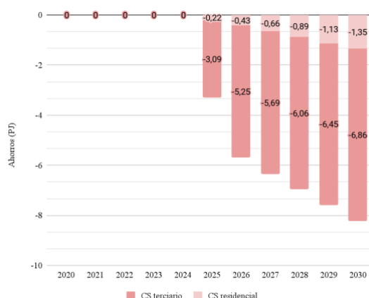
Gráfica 38. Reducción de demanda esperada de las medidas de eficiencia energética por medidas de construcción sostenible.
