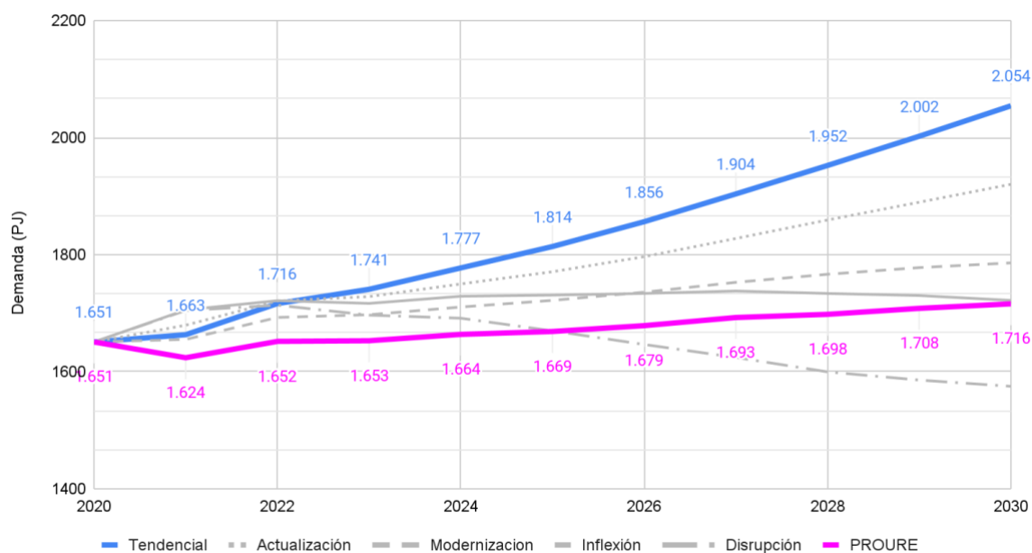
Gráfica 3. Comparación del consumo estimado para el escenario PAI-PROURE 2021-2030 frente al escenario tendencial y los del PEN 2020-2050
