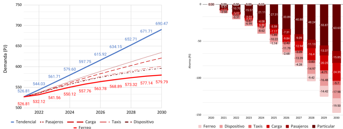
Gráfica 15. Reducción de demanda esperada de las medidas de eficiencia energética en el sector transporte en el PAI-PROURE
