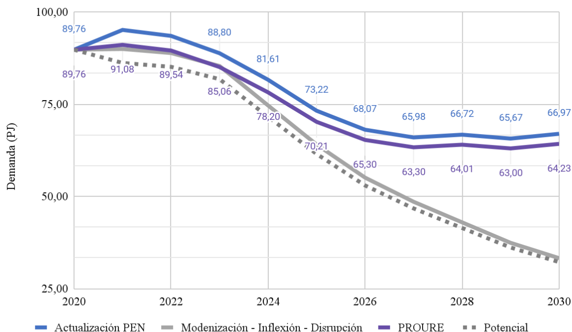
Gráfica 30. Comparación de escenarios de consumo energético para el sector hidrocarburos
