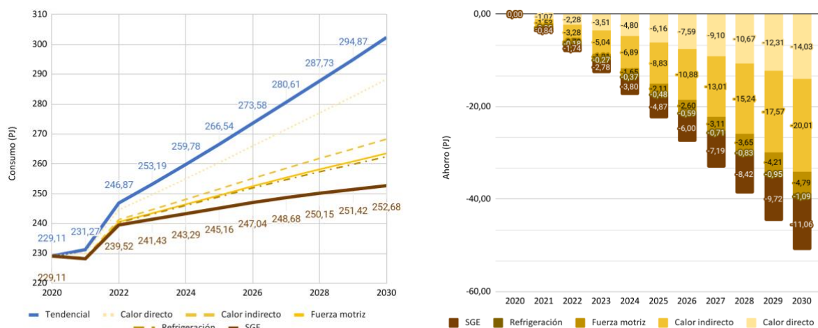
Gráfica 19. Reducción de demanda esperada de las medidas de eficiencia energética en el sector industrial en el PAI-PROURE
